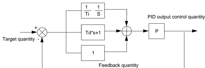
شکل 1-5-5 نمودار کنترل فرآیند PID
